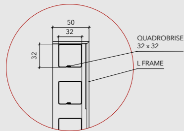
CORTE C
