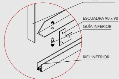
DETALLE CONJUNTO B
