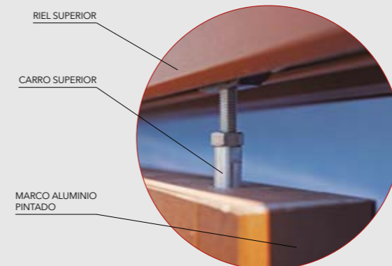
DETALLE SUPERIOR
