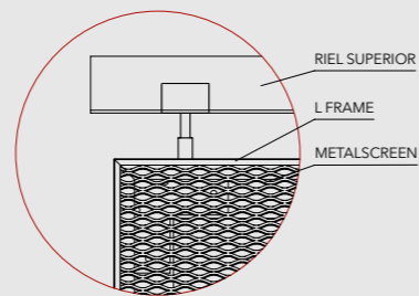
DETALLE A
