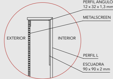
CORTE D
