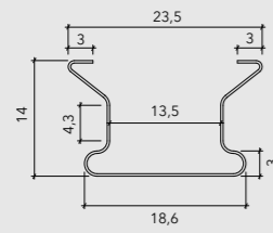
JUNTA RAS
