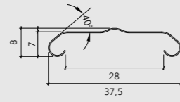
ANCLAJE SOPORTE
