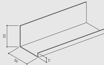
PERFIL MULLION
