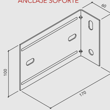
ANCLAJE SOPORTE
