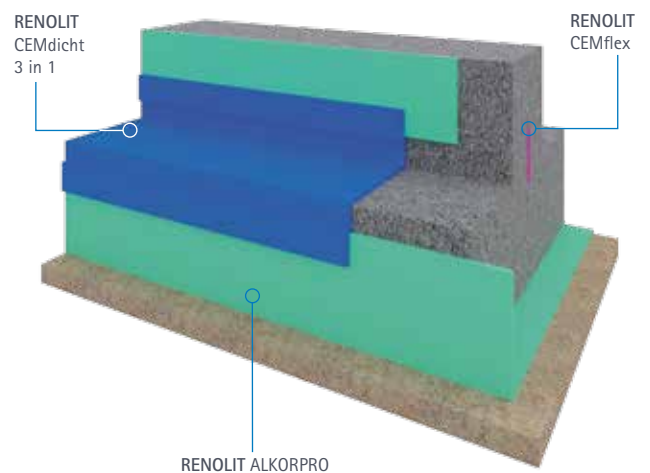
Zapatatas
