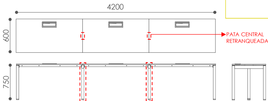
PLANIMETRÍA EN MILIMETROS
