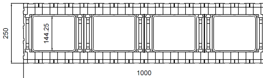
VISTA SUPERIOR
