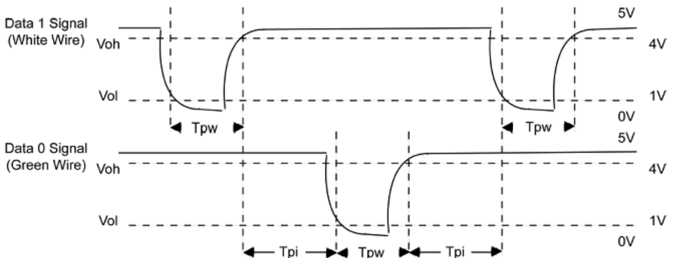
Figura 1: Diagrama Secuencial
