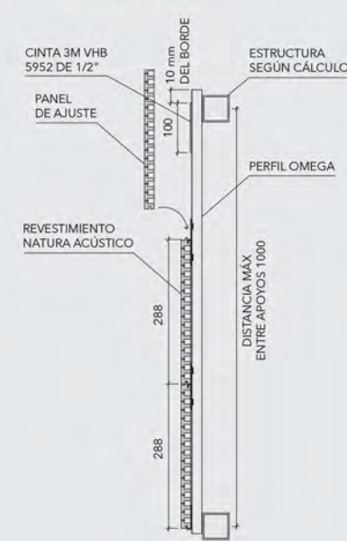
CORTE A-A
