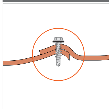
Detalle fijaciones de traslape
