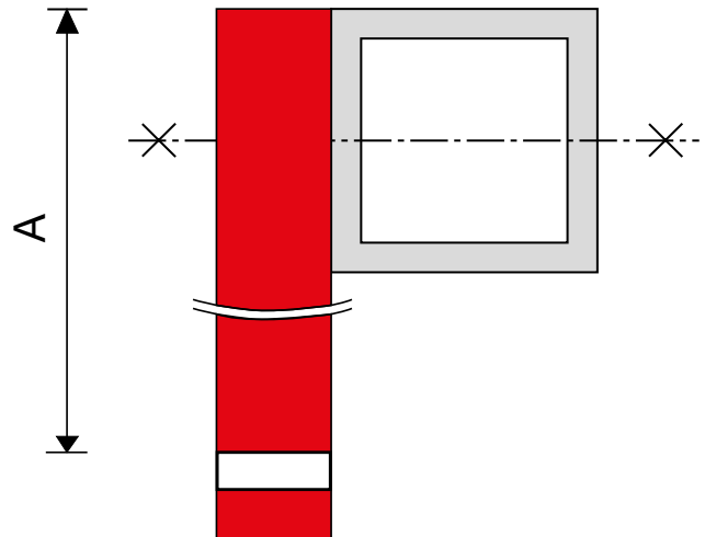
CORTE VERTICAL DEL PERFIL DEL DINTEL SOBRE LA PUERTA
