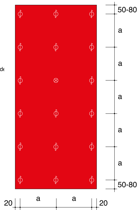
FIG. 3 TRAMO DE PLACA DOBLE
