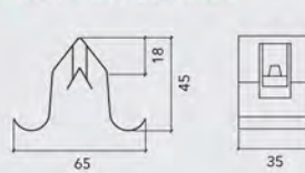
CLIP ANTISÍSMICO
