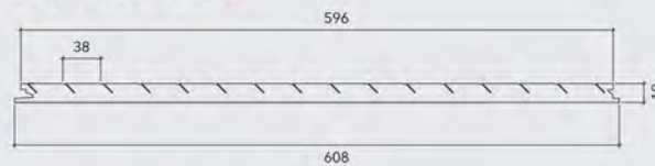
SECCIÓN SUPERIOR
