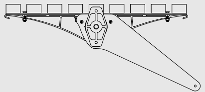
CORTE A-A
